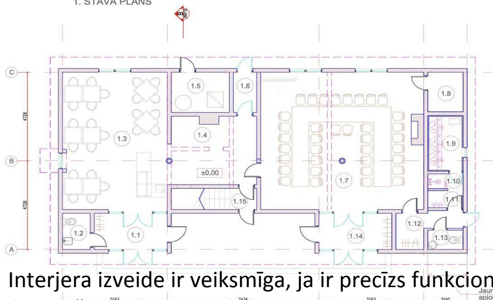
1. STĀVA PLĀNS
