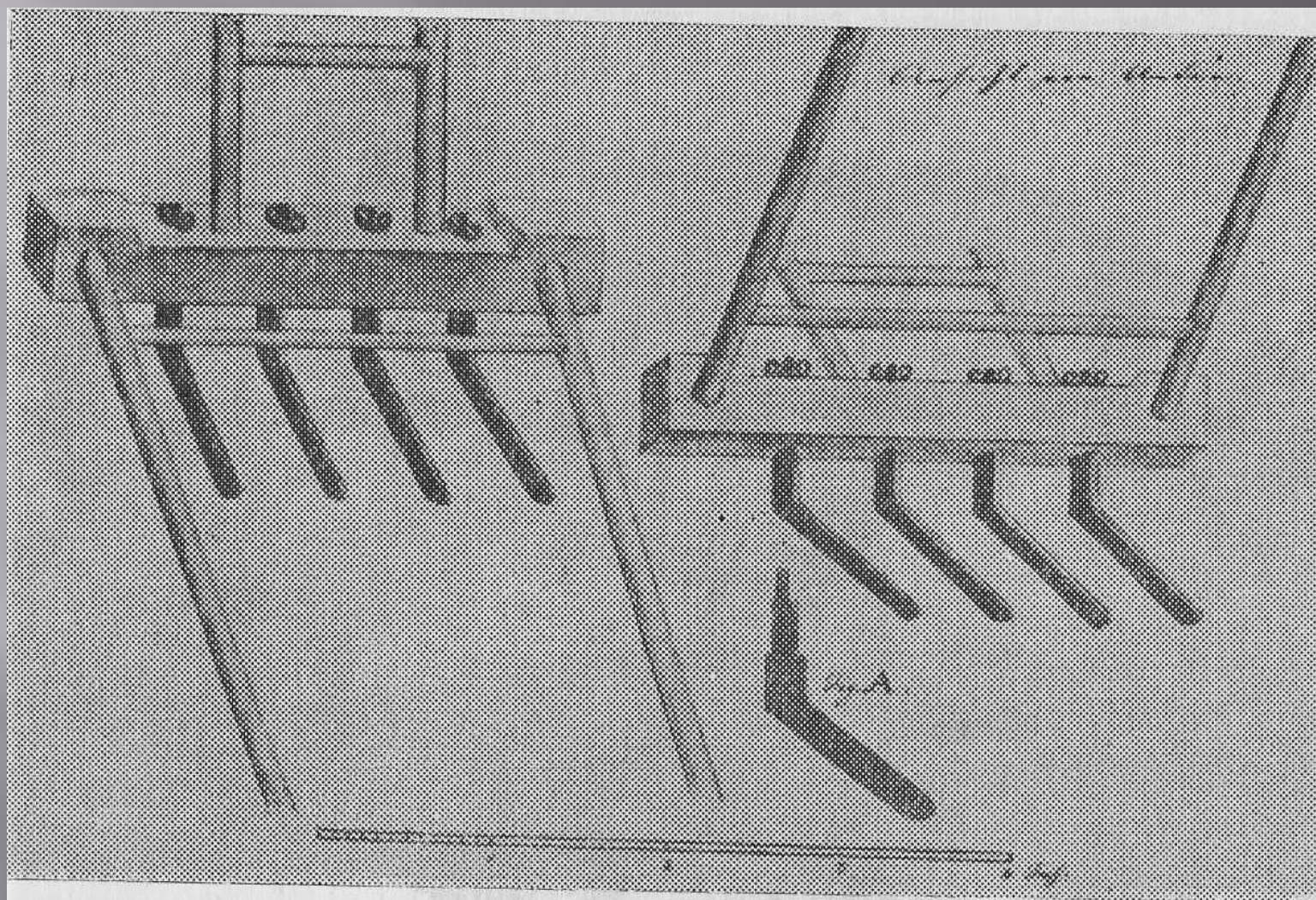
J. Krēsliņa kultivators 1831. gada 25. septembrī
